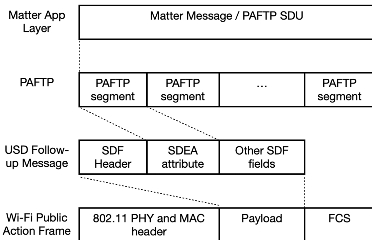
Figure 30. MATTERoPAF: Matter Message / PAFTP layering
